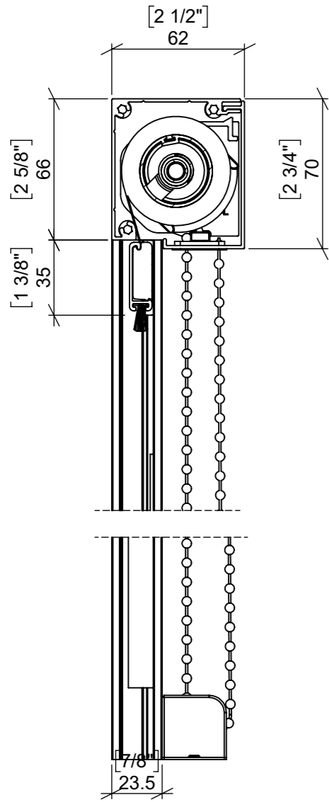
SECTION A-A
