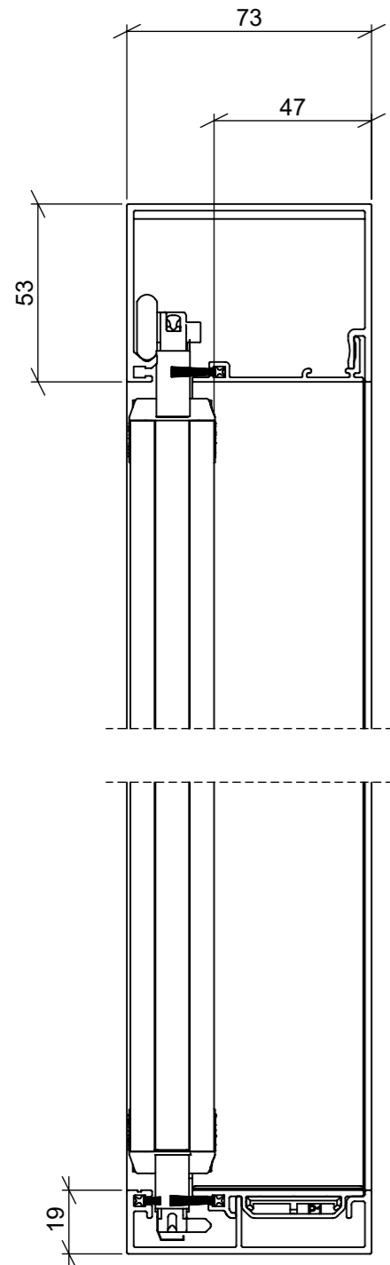
SECTION A-A
