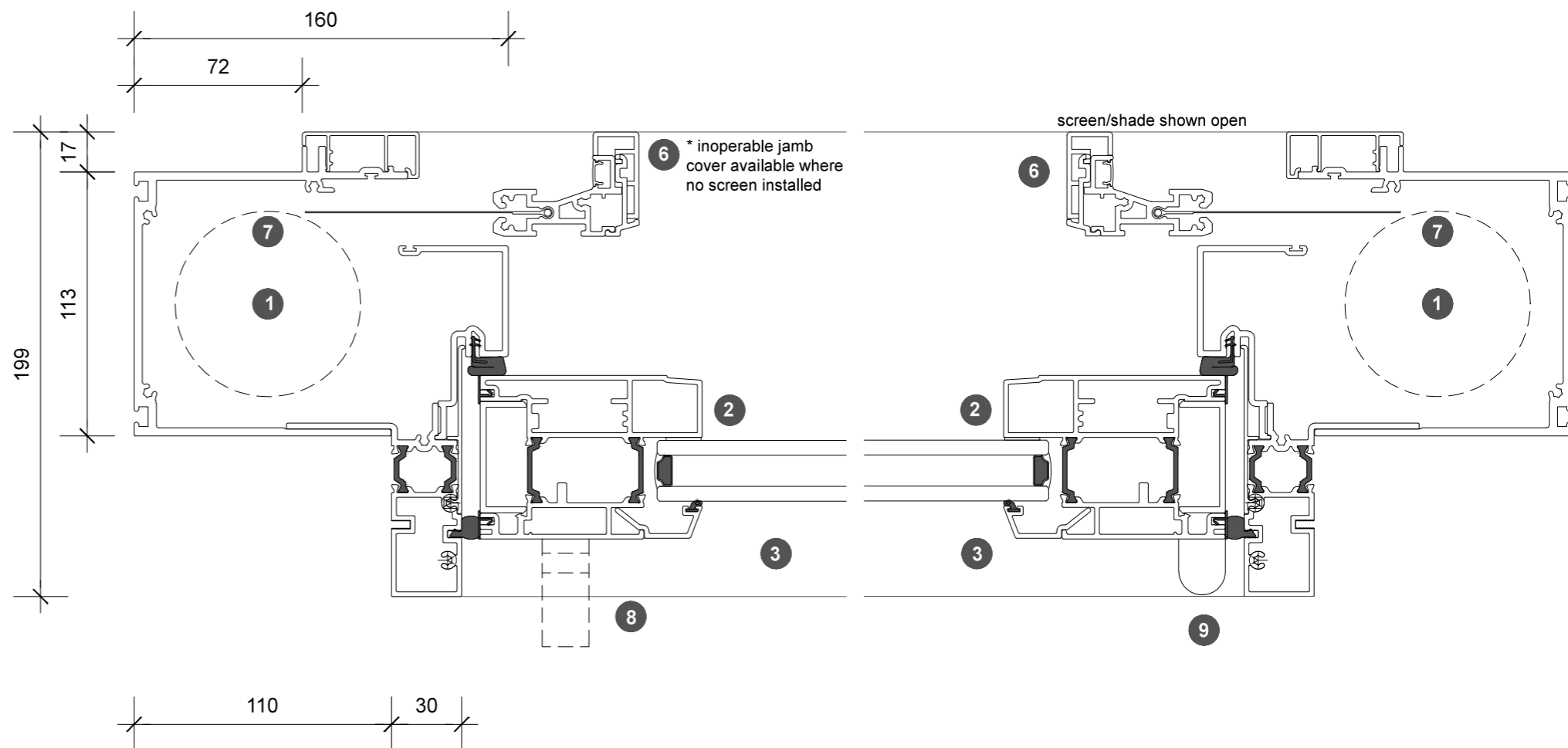
1. jamb detail
